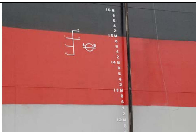
船的載重線
