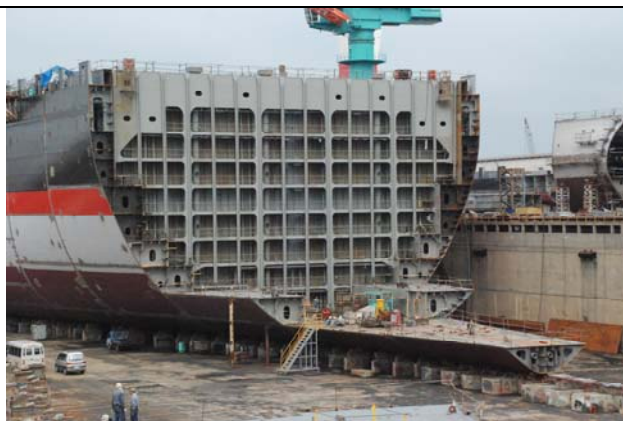
建造中的貨櫃船
