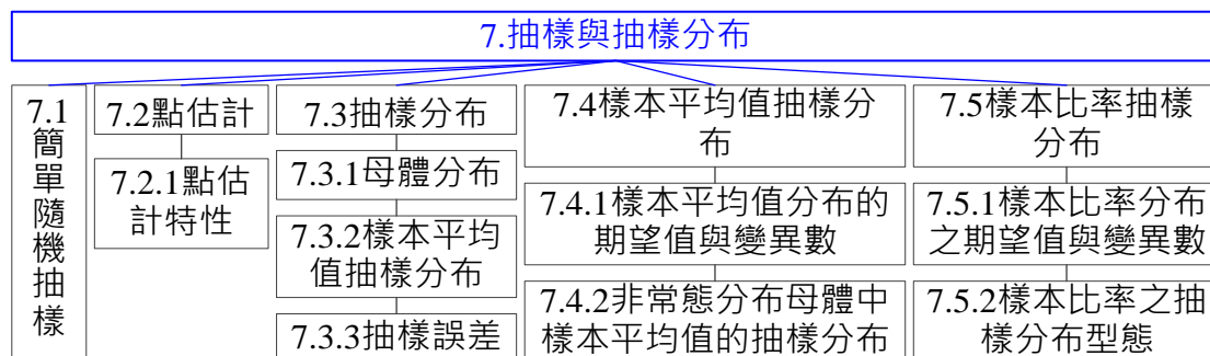
章節結構圖
